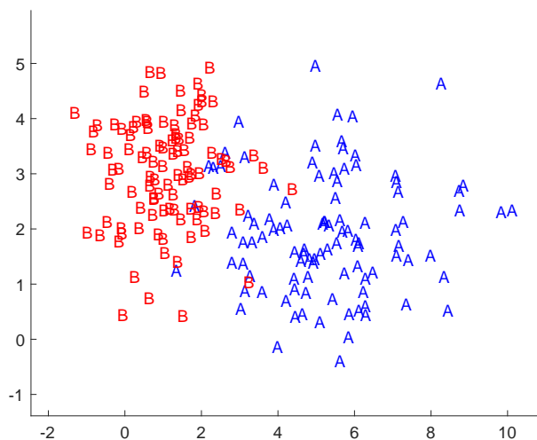
圖 5: 繪製群組資料
