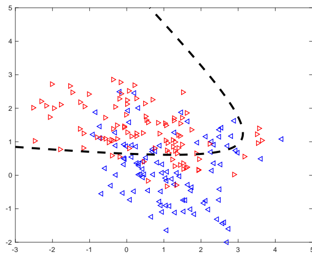
圖 10: 加廣型迴歸的非線性群組分界線
