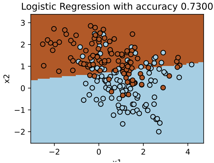
圖 11: 羅吉斯迴歸的準確率：資料來源 la_3.txt
