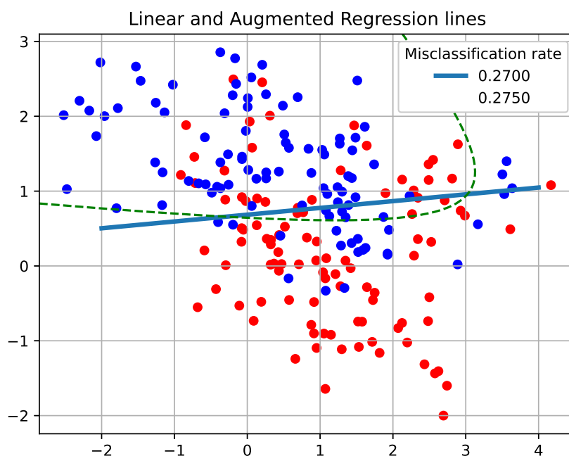
圖 9: 線性與加廣型迴歸的錯判率
